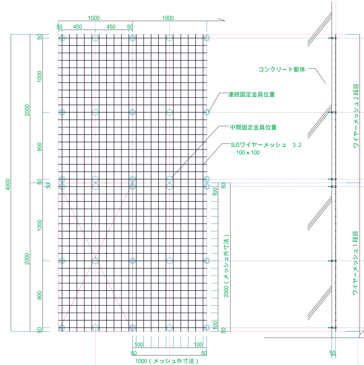
正面図 S=1/25
